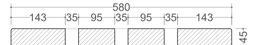
SEZIONE
