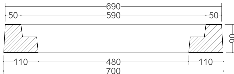
SEZIONE
